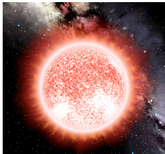
ANTARES Corazón del Escorpión, Rival de Marte Estrella Gigante Roja Magnitud: 1 Constelación: ALFA ESCORPIO
